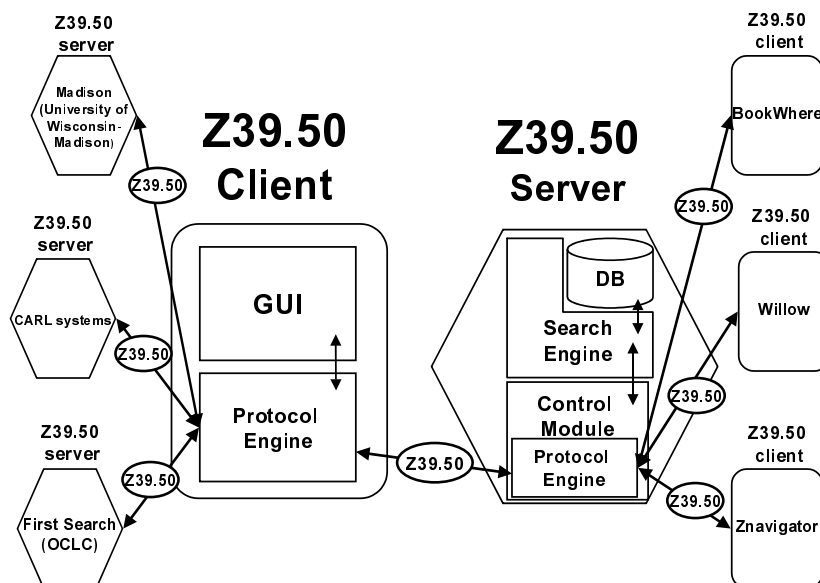
図 2.1 Z39.50 の全体像
