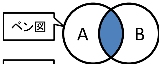
論理積
