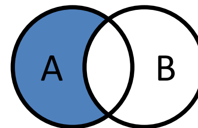
論理差
