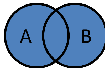
論理和
